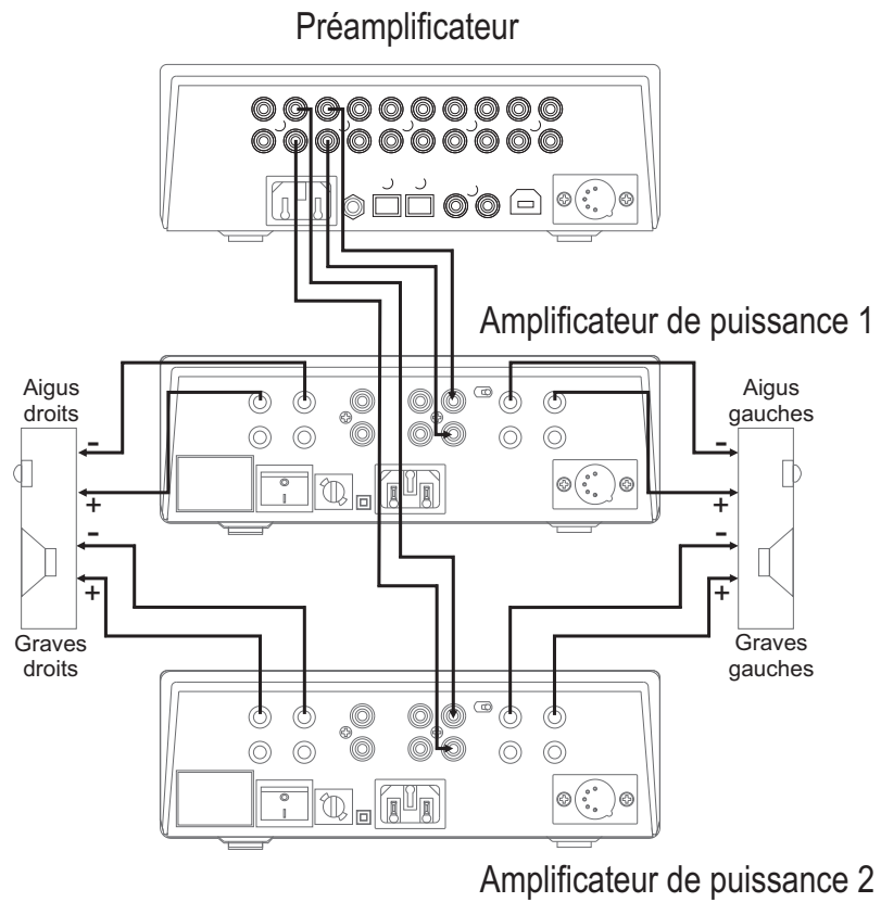
Raccordement d'un système d'enceintes bi amplifié à un préamplificateur
